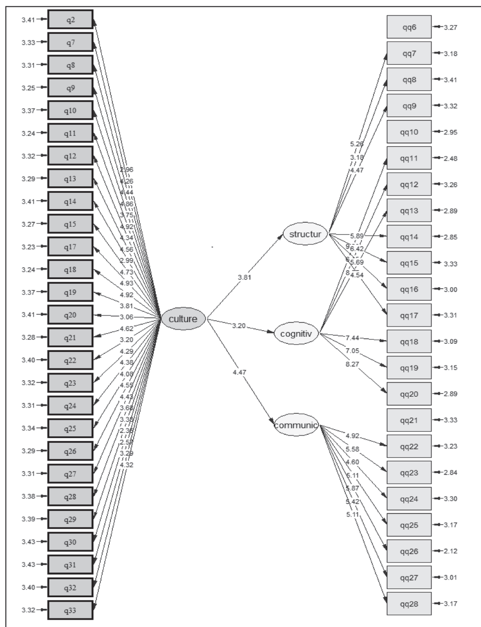
شکل ۲: مقادیر تی (سطح معناداری) مدل تحقیق
